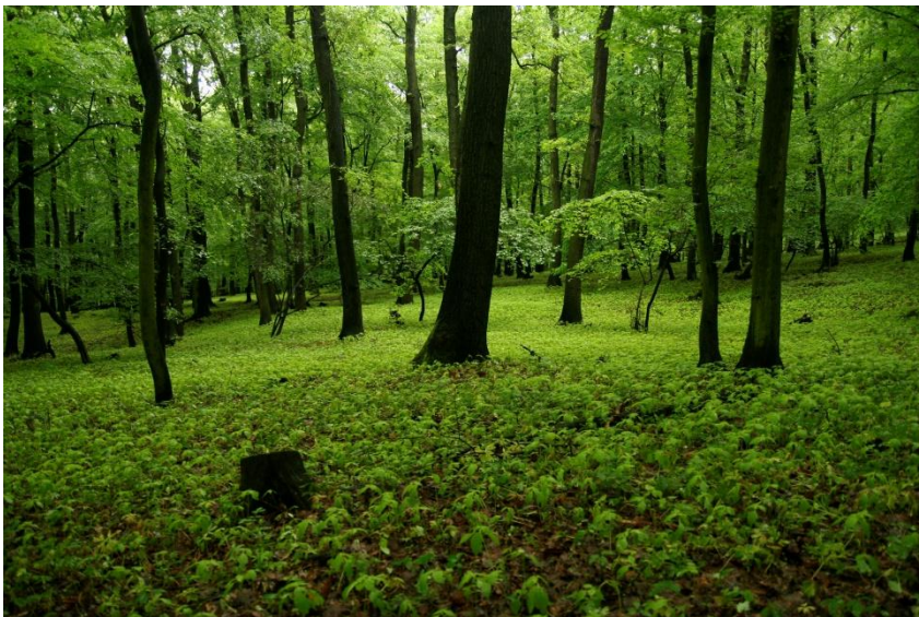
Obr. 4. Netýkavka malokvětá, druh, který ze vzduchu mapovat nelze.
