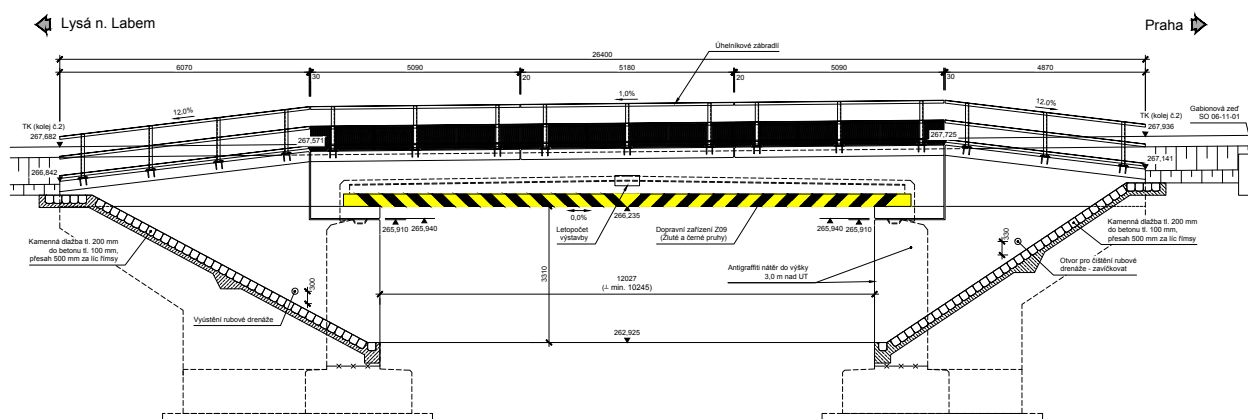
SO 06-20-05 MSTĚTICE - PRAHA HORNÍ POČERNICE ŽELEZNIČNÍ MOST V EV. KM 19,503 PODÉLNÝ ŘEZ MOSTEM M 1:50
