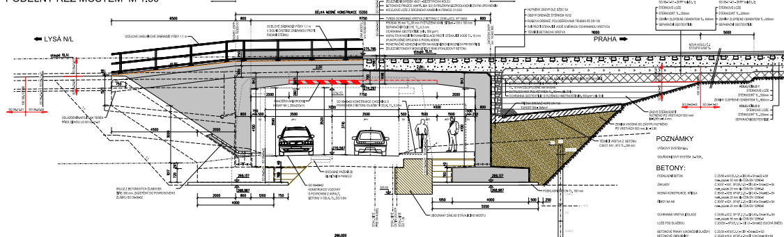
SO 06-20-05 MSTĚTICE - PRAHA HORNÍ POČERNICE ŽELEZNIČNÍ MOST V EV. KM 19,503 PODÉLNÝ ŘEZ MOSTEM M 1:50
