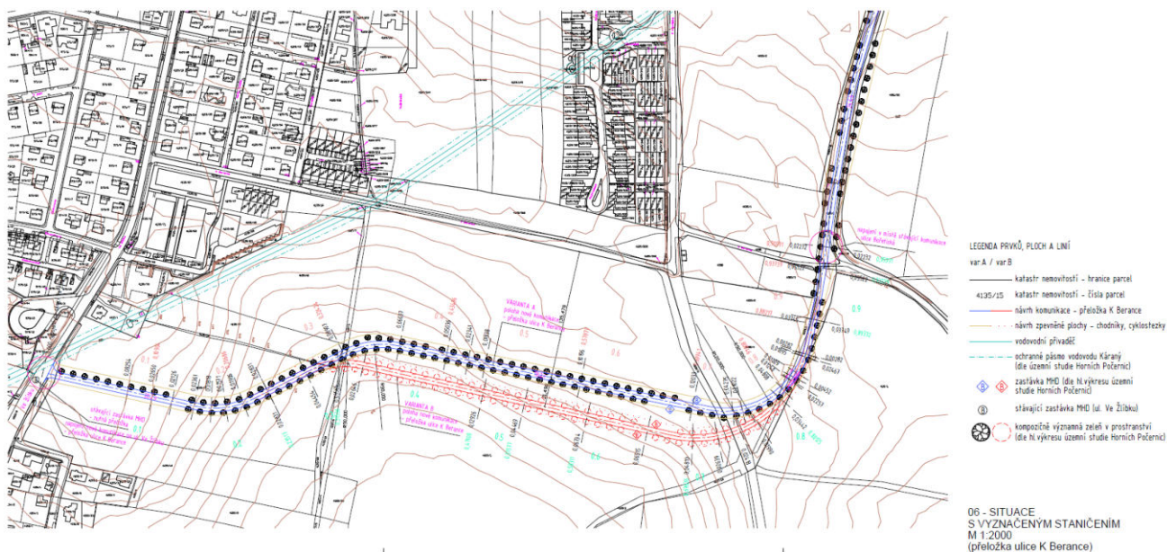
Podkladová studie pro návrh změny ÚPn HMP Z 2872/00 „Přeložka komunikace K Berance“ - výkres č. 06_Situace s vyznačeným staničením
