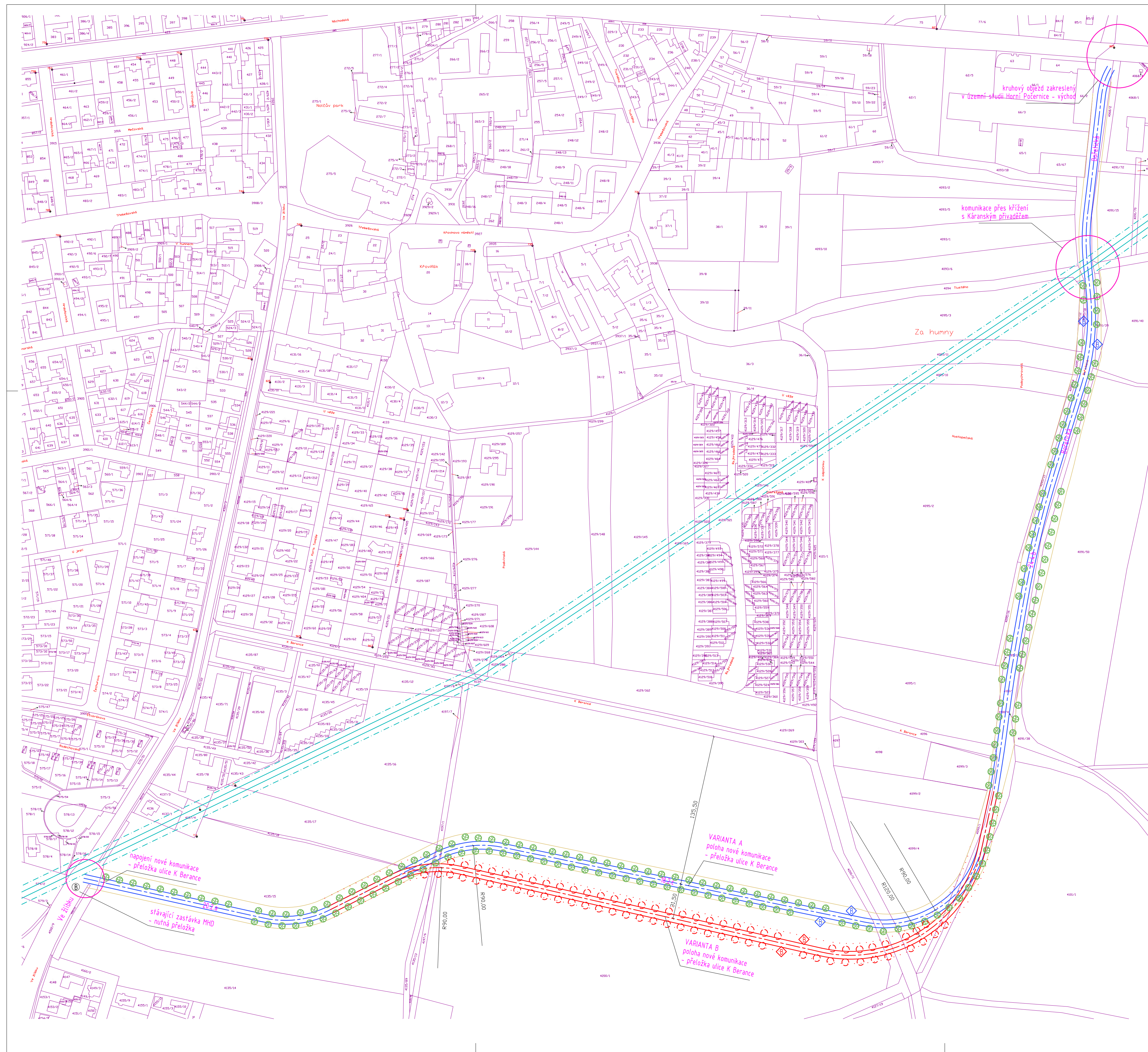
01 - SITUACE NA PODKLADU KATASTRÁLNÍ MAPY M 1:2000 (přeložka ulice K Berance)
