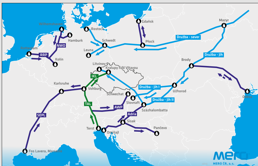
Schéma hlavních evropských ropovodů včetně tras TAL, IKL a Družba, které propojují Českou republiku s evropskou ropnou infrastrukturou a umožňují diverzifikaci dodávek ropy
